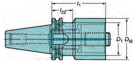
C6-390.272-40 085
