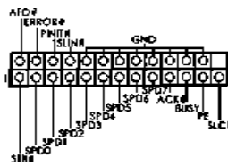
打印机端口接针 (25 针 LPT1) (见第 2 页第 22 项)
