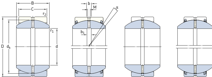
GEZ..ES
