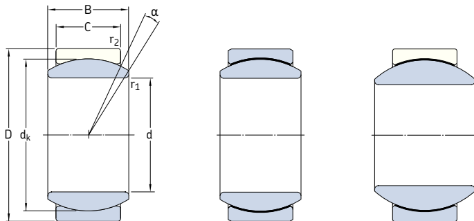
GE .. C
