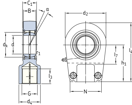
SI(L)R..ES
