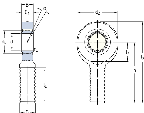
SA(L).. C
