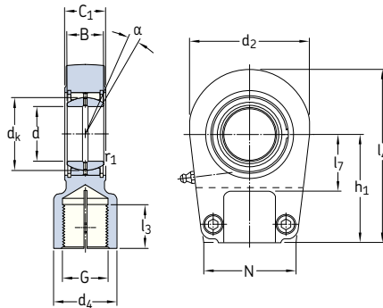
SI(L)R..ES
