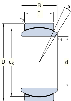
GE .. TXGR
