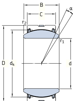
GEZ .. TXA-2LS
