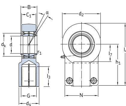
SI(L)QG..ES
