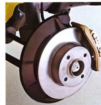
Vorn hat der Audi 50 große Schwimmsattel-Scheibenbremsen.
