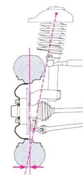
Die Audi 50-Vorderachse mit spurstabilisierendem Lenkrollradius. Die Lenkachse (gestrichelte Linie) endet hier nicht wie bei anderen Vorderradaufhängungen innerhalb (positiver Lenkrollradius) oder genau in der Radmittelebene (Lenkrollradius null), sondern außerhalb der Radmittelebene (spurstabilisierender Lenkrollradius).
