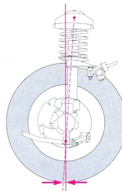
Durch den Nachlaufversatz der Federbeine wird ein besonders gutes Sturz- und Lenkverhalten der Vorderräder sowie ein kleiner Wendekreis erreicht.
