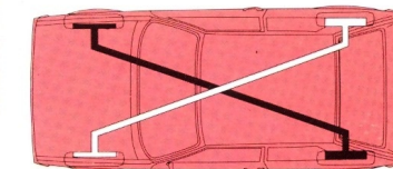
Die zwei Bremskreise des Audi 50 sind über Kreuz angeordnet. So wird bei Ausfall eines Kreises noch je ein Vorder- und Hinterrad gebremst.
