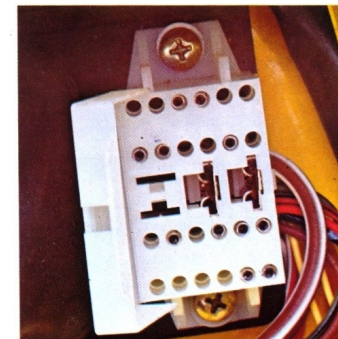
Die Diagnose-Steckdose des Audi 50 für die Computer-Diagnose.
