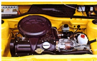
Der robuste Audi 50-Motor ist sehr leistungsstark.
