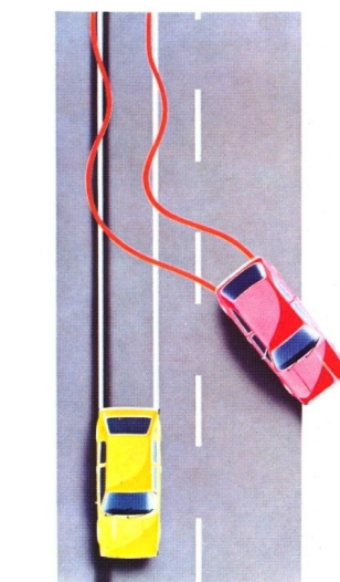
Bei diesem Bremstest auf einer Asphaltstraße, die auf einer Seite mit einer Ölspur versehen ist, zieht das Auto mit konventioneller Bremsanlage beim Bremsen schief und bricht aus. Der Audi 50 mit Lenkstablem Bremssystem bleibt spurgenaue gerade.
