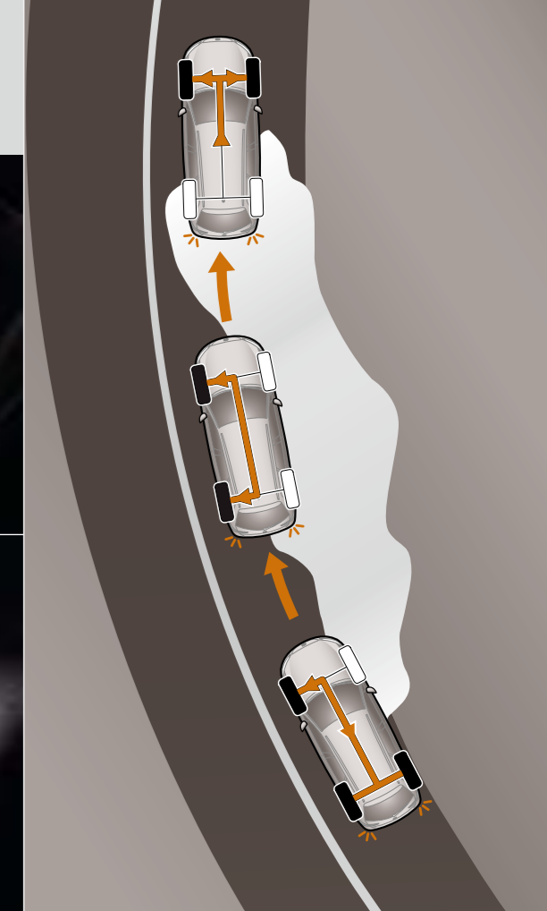
El Sistema de Control de Tracción (TCS) traza las curvas sin perder potencia. El Programa Electrónico de Estabilidad (ESP) controla y ajusta la situación de neumáticos, frenos, acelerador y volante.
