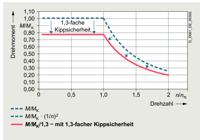
Überlastmomentkennlinie SIMOTICS GP/SD VSD10-Linie
