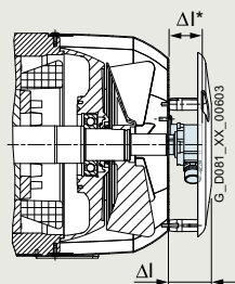
Bild 2 Drehimpulsgeber (auf Haube), Kurzangaben G04/G05/G06/G11/G12 [ G11, G12 standardmäßig mit Schutzdach]
