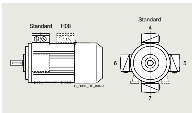
Lage des Anschlusskastens mit den entsprechenden Ziffern an der 16. Stelle der Artikel-Nr.
