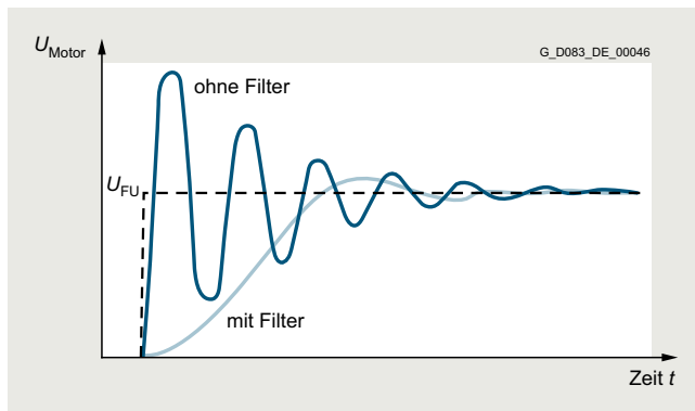
Typischer Verlauf der Umrichterspannung U_{FU} und der Motorspannung U_{Motor} am PWM-Umrichter (Umrichter ohne und mit Ausgangsfilter)
