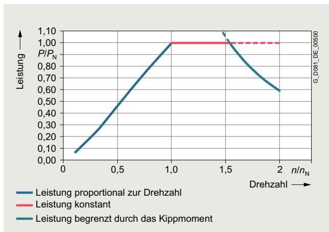
Grenzleistung SIMOTICS GP/SD VSD10-Linie eigengekühlt
