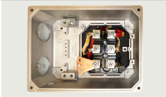
Anschlusskasten Typ TB1L10 – Kurzangabe R50
