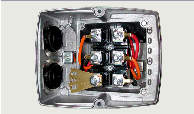
Anschlusskasten Typ TB1L00
