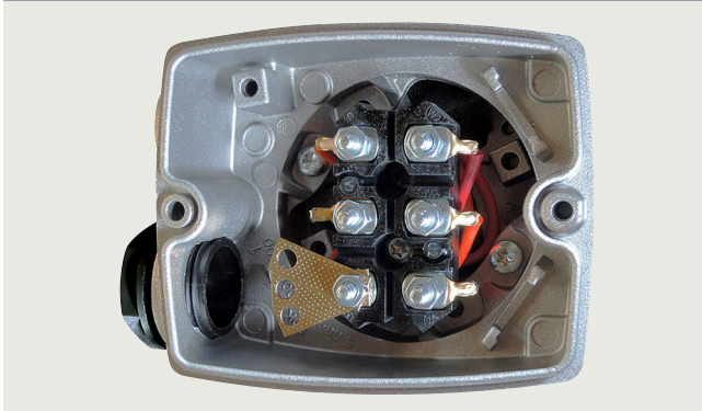
Anschlusskasten Typ TB1F00, TB1H00, TB1J00
