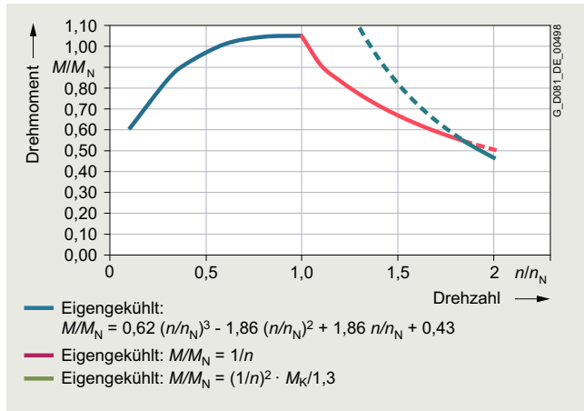
Grenzmomentkennlinie SIMOTICS GP/SD VSD10-Linie eigengekühlt
