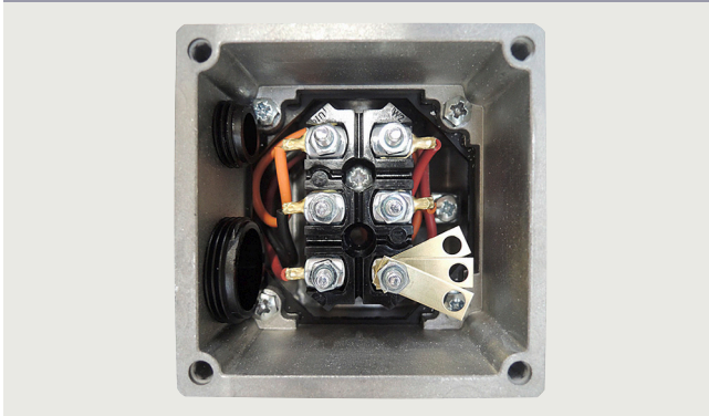
Anschlusskasten Typ TB1E00
