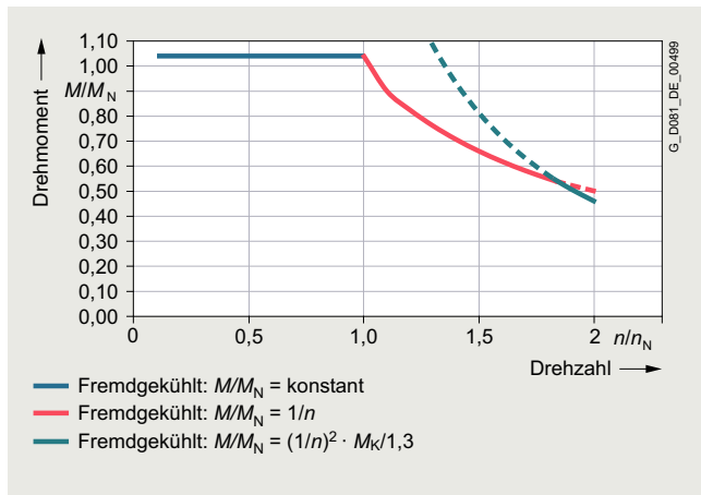
Grenzmomentkennlinie SIMOTICS GP/SD VSD10-Linie fremdgekühlt
