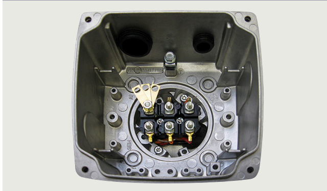
Anschlusskasten Typ TB1F10, TB1H10, TB1J10 – Kurzangabe R50
