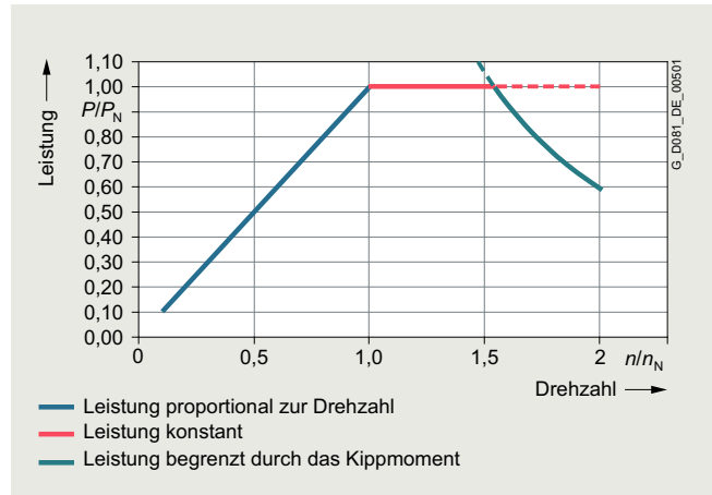
Grenzleistung SIMOTICS GP/SD VSD10-Linie fremdgekühlt
