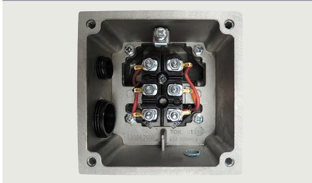
Anschlusskasten Typ TB1E10 – Kurzangabe R50
