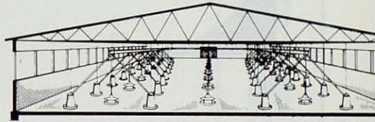
Detalle de una instalación de comedero automático PUIG COLGANTE y BEBEDEROS DRINKEV. Se pueden instalar 1, 2 y 3 filas de tolvitas PLASTIC PUIG o PUIG-MATIC, filas se doblan con las ventajas de distribución de pienso retorno.
