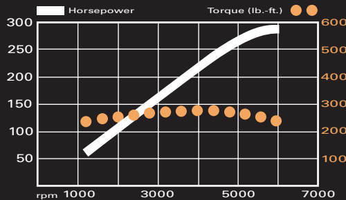
4.2L Vortec 4200 I-6
